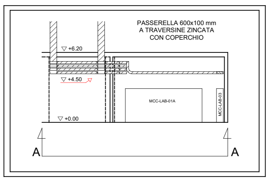
PARTICOLARE PASSERELLE (sez. A-A e B-B)
