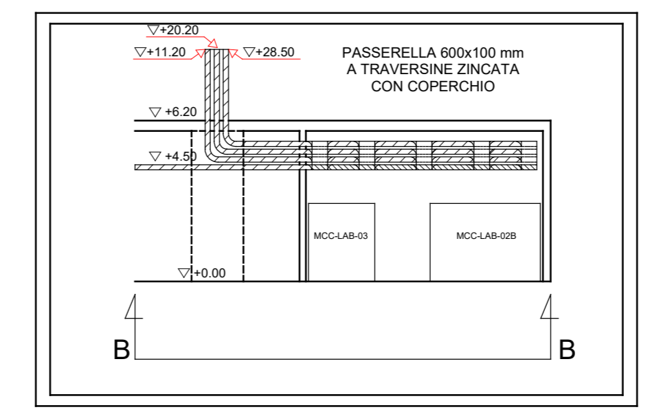
PARTICOLARE PASSERELLE (sez. A-A e B-B)
